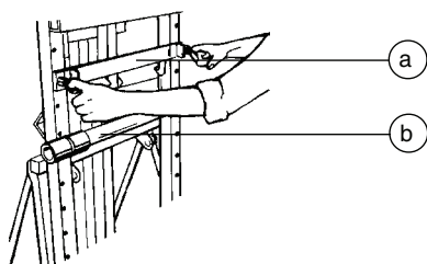
a aanslagbeugel b draaistang voor laden
