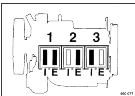
Afb. 193: Krukasstand 2
