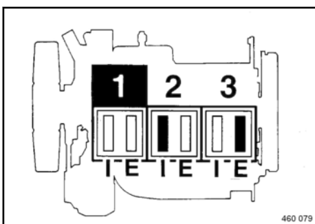
Afb. 191: Krukasstand 1
