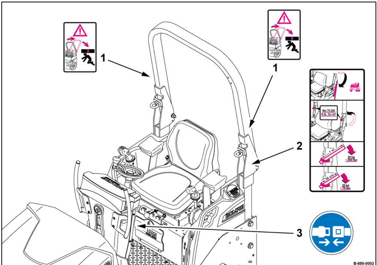
Afb. 10: Bebording klap-ROPS
