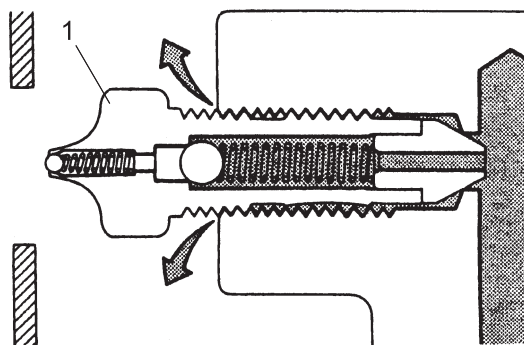
Details van een Sectie (Vet Aftappen)
