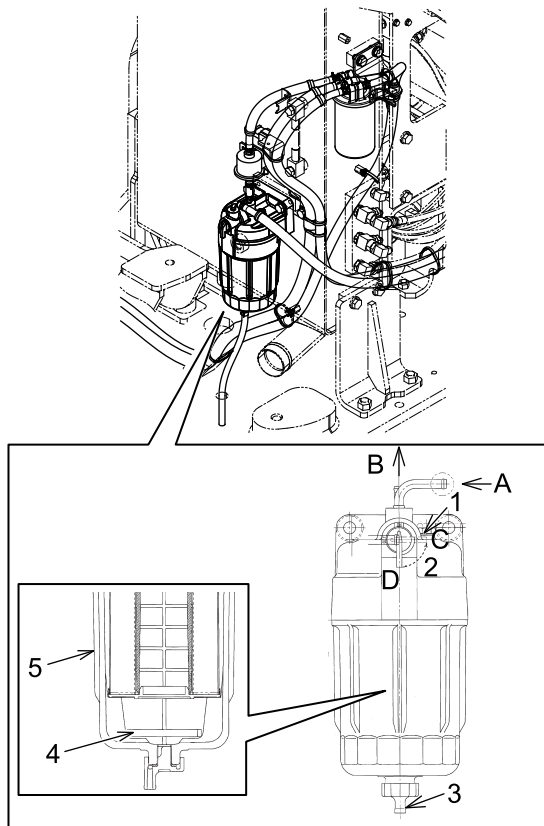
Brandstofvoorfilter
