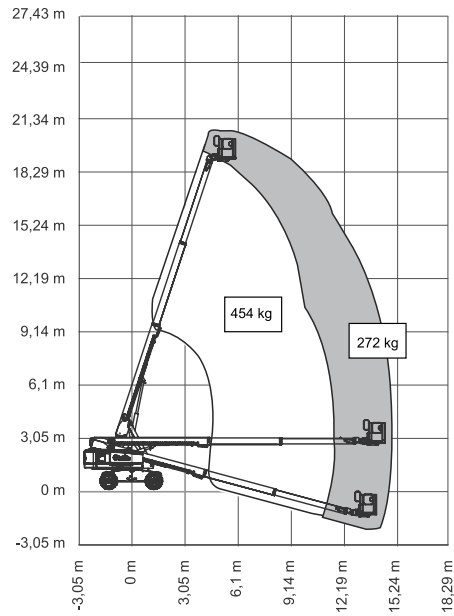
Diagram werkbereik S-65 HF
