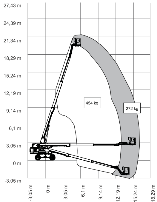
Diagram werkbereik S-65 HF
