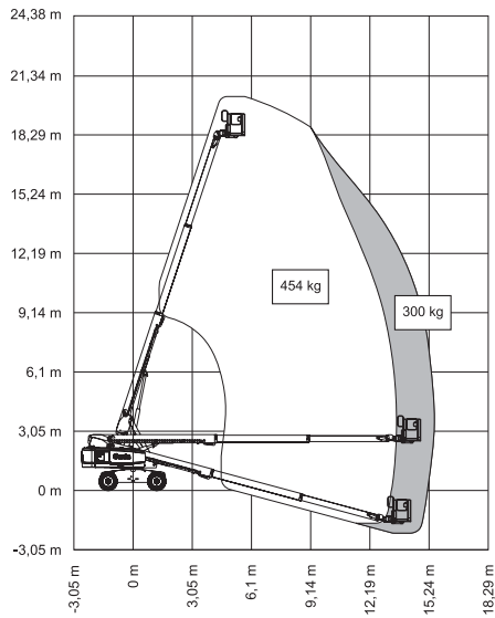
Diagram werkbereik S-65 XC en S-65 TRAX
