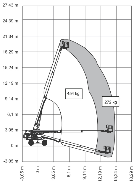
Diagram werkbereik S-60 HF
