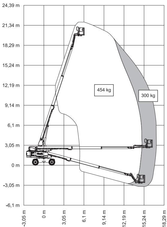
Diagram werkbereik S-60 HF
