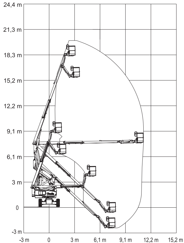
Diagram werkbereik Z-60/37DC en Z-60/37FE
