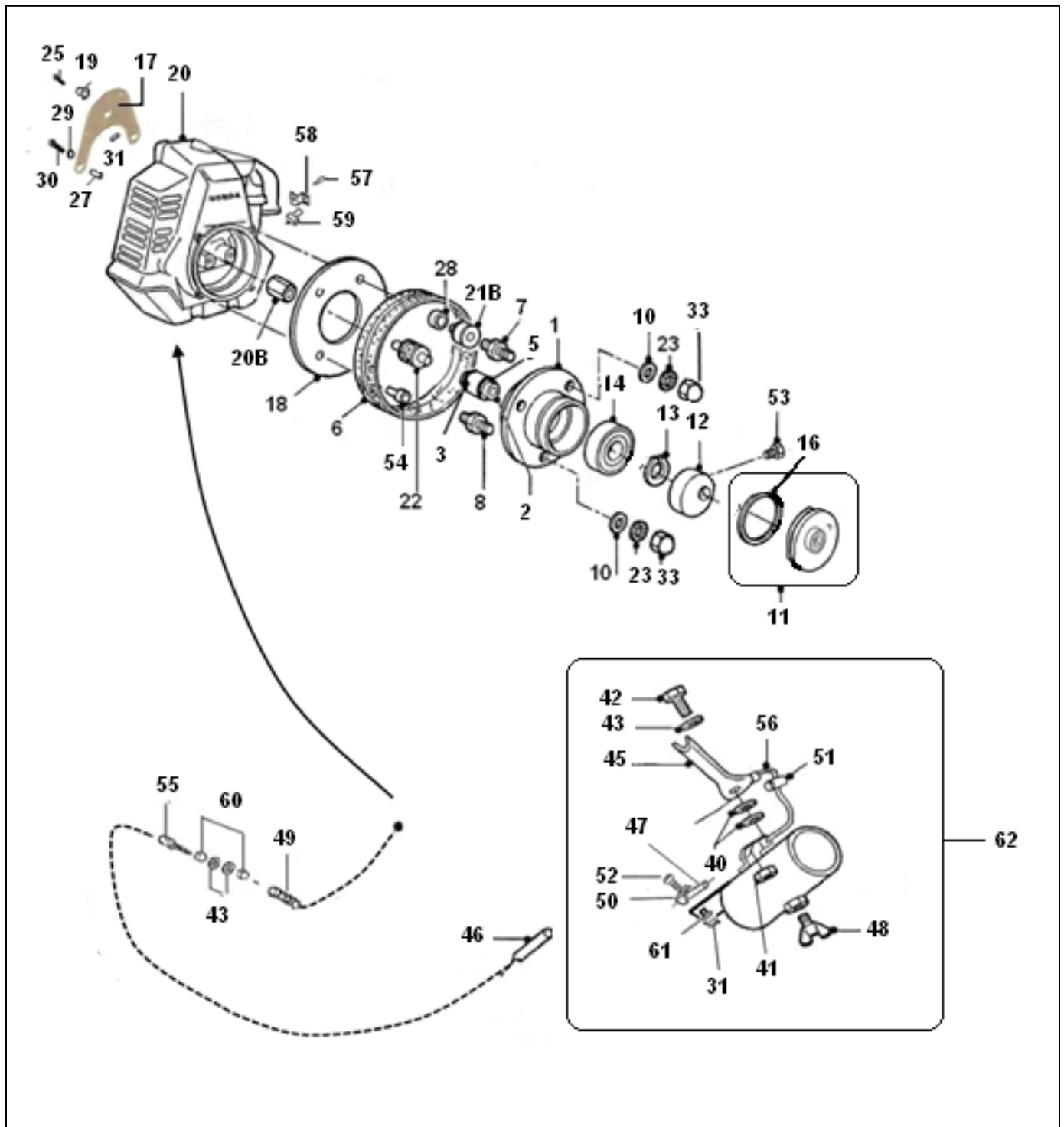
Fig. 12: Aandrijfmotor en excentriek dubbellager K-150 B
