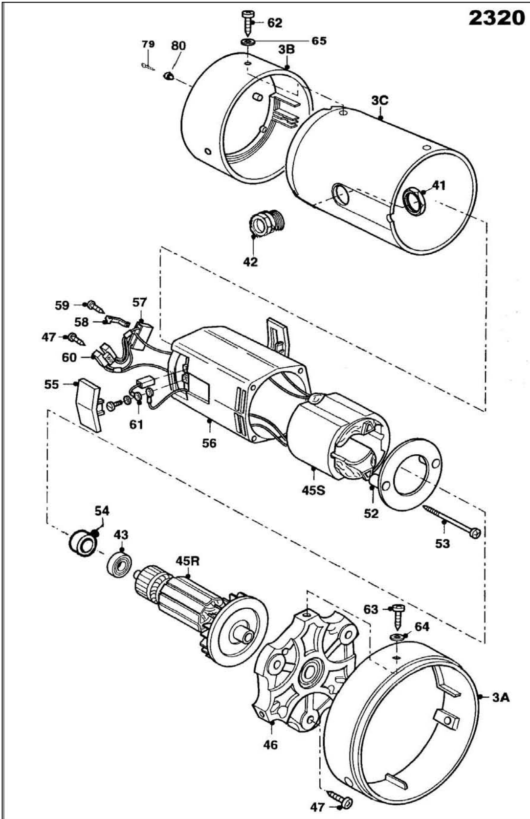
Fig. 10: Aandrijfmotor K-150 E, ER
