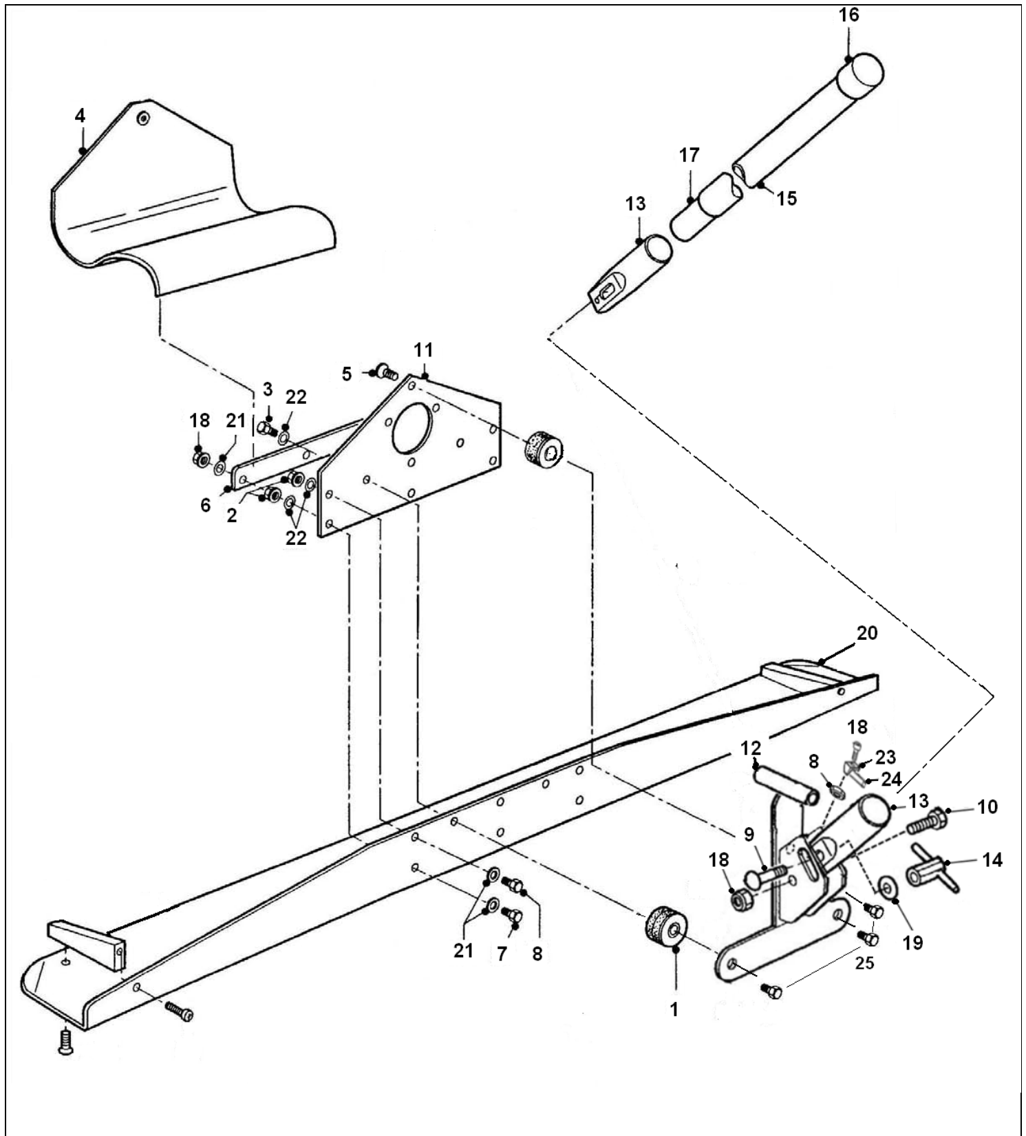
Fig. 9: Frame K-150 E, ER, B
